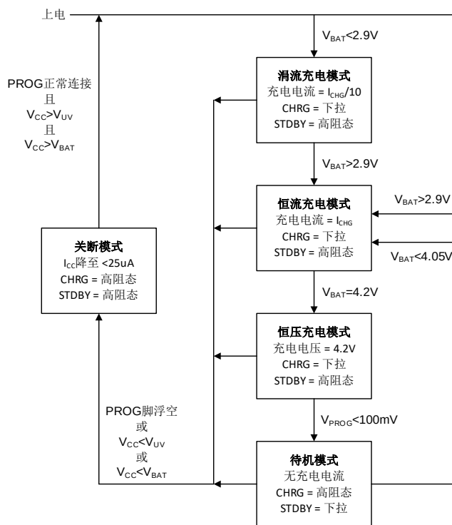
图2 典型充电循环的状态图
