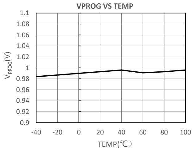
PROG引脚电压 vs 温度
