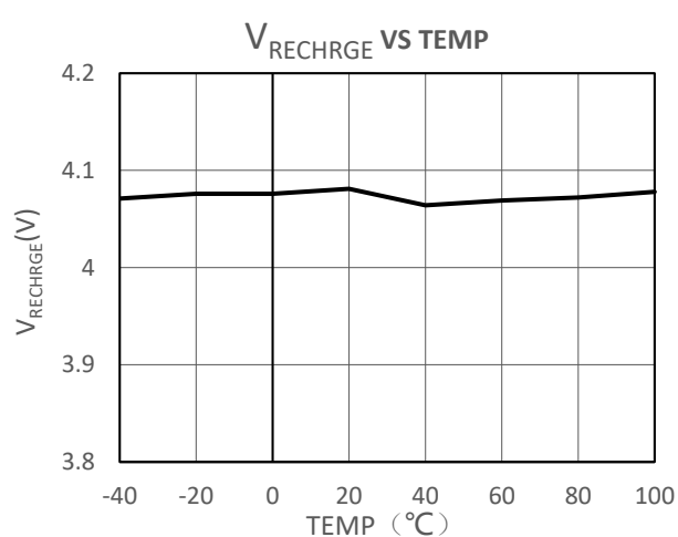
再充电电压 vs 环境温度
