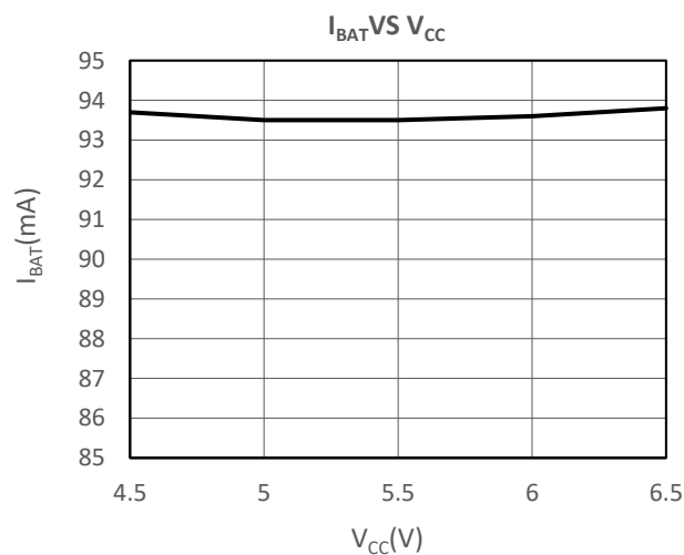
充电电流 vs 电源电压 ( R_{\text{PROG}}=10\text{K}\Omega )
