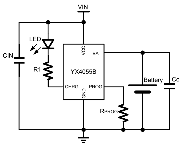
图 4. 典型应用电路
