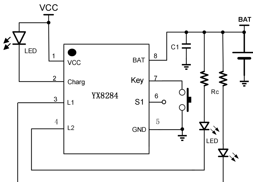
图 2. 典型应用电
