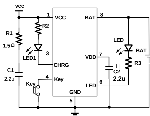
图 1. 典型应用电路
