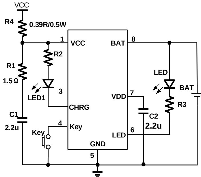
图五. 大电流充电时减少芯片发热量的应用电路
