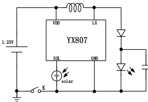
图 6. 推荐接法 2
