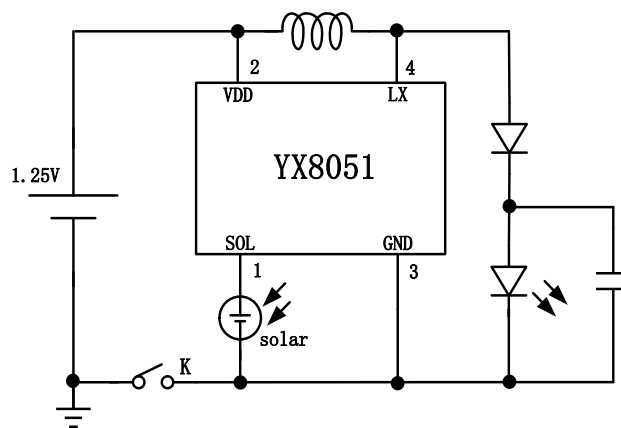
图 6. 推荐接法 2
